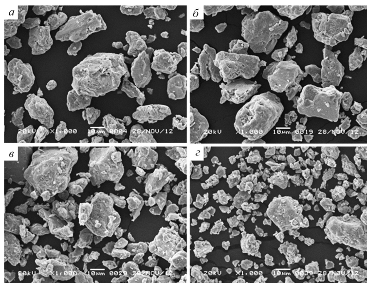
Рис. 2. Морфология частиц порошка Cu–13 мас.% Al в зависимости от продолжительности МА ( а , б , в , з – 3, 6, 9, 12 мин соответственно), \times 1000
