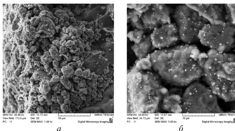
Рис. 6. СЭМ-фотографии мембранного слоя Cu–13 мас.% Al на титановой подложке (12 мин МА): а – ×1000; б – ×5000
