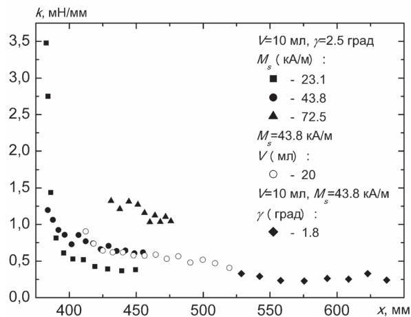
Рис. 5. Зависимость коэффициента упругости капли от ее положения в канале
