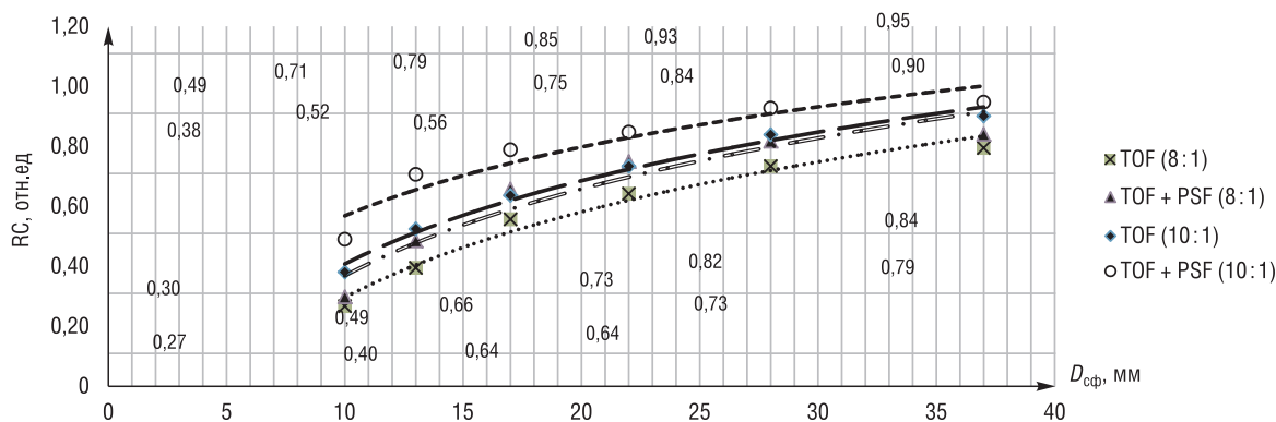
Рис. 1. Зависимость коэффициента восстановления от размеров сферы
